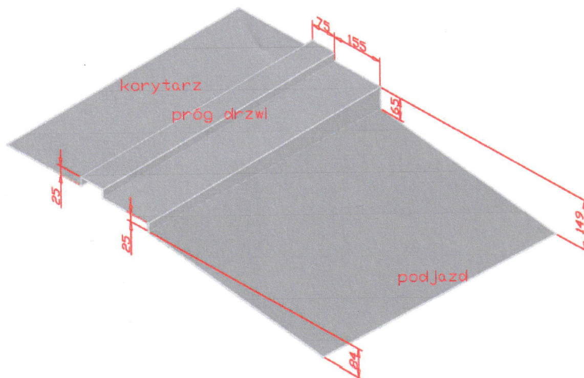
Rysunek nr 1. Wymiary progu budynku
